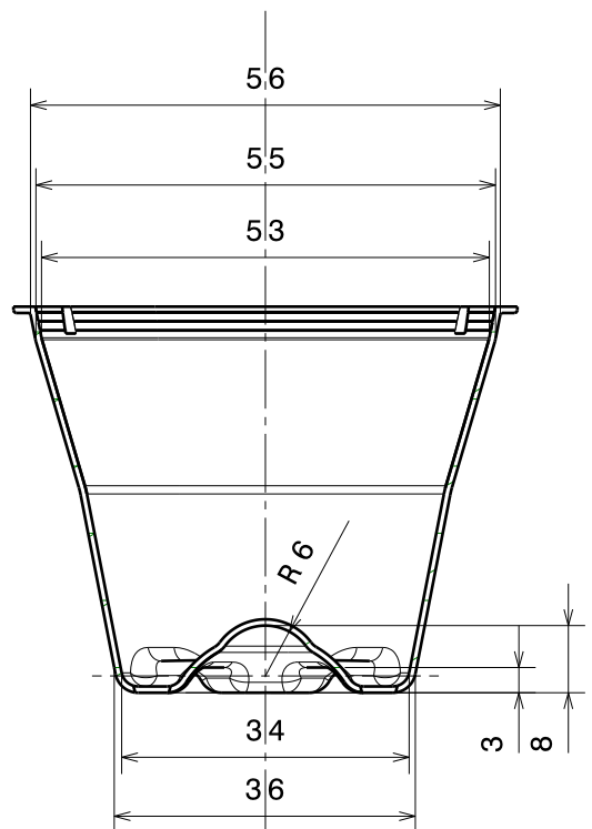
Section view A-A Scale: 1:1
