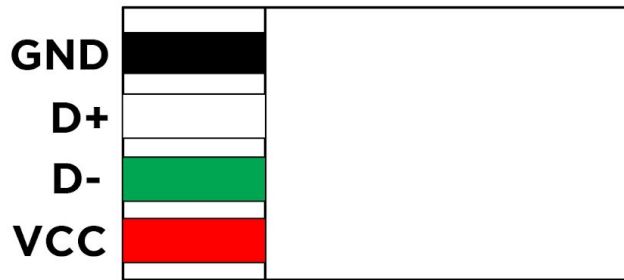
USB-A
