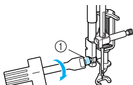
① Vis du support de pied-de-biche
