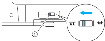
① Levier d'entraînement par griffe (vu depuis l'arrière de la machine) ▶ Les griffes d'entraînement sont abaissées.
