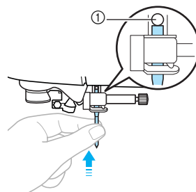
① Butée d'aiguille
