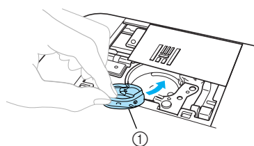
① Compartiment à canette
