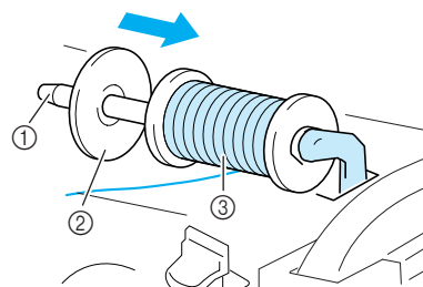
① Porte-bobine supplémentaire ② Couvercle de bobine ③ Bobine de fil
