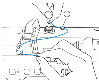
① Guide-fil
