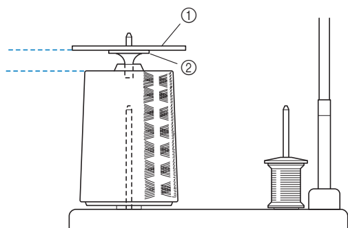
① Couvercle de bobine ② Base de couvercle de bobine
