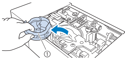
① Boîtier de canette
