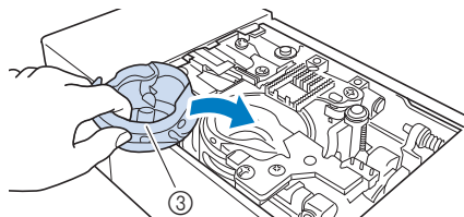
① Marque ▲ sur le boîtier de canette ② Marque ● sur la machine ③ Boîtier de canette
