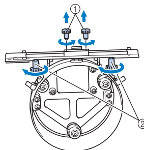
① Vis supérieures ② Vis inférieures
