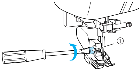
① Vis du support de pied-de-biche
