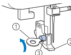
① Tournevis en forme de disque ② Support du pied-de-biche ③ Vis du support de pied-de-biche
