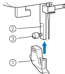
① Support du pied-de-biche ② Barre du pied-de-biche ③ Vis du support de pied-de-biche
