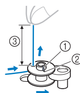
③ 7-10 cm (3 à 4" / pouces)
