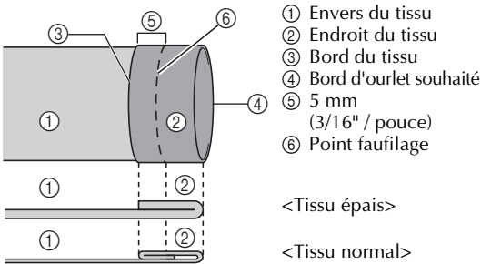
<Vu de côté>
