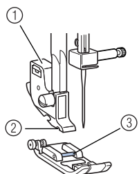
① Support du pied-de-biche ② Talon ③ Épingle
