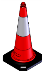
PARK-DH-PE-2 ΠΛΑΣΤΙΚΟΣ ΚΩΝΟΣ 75 cm με βαριά λαστιχένια βάση Βάση: 38x38cm (3.3 kg)
