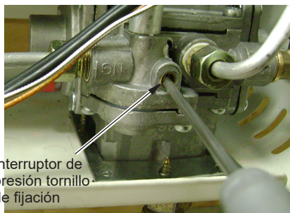
Figura 30 - Interruptor de presión del regulador de gas (Interior de la parte inferior del gabinete del calentador)
