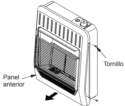
Figura 5 - Desmontaje del panel anterior
