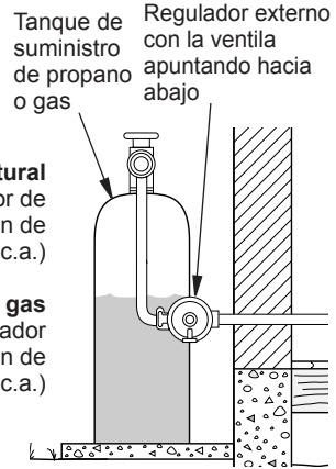
Figura 13 - Regulador externo con la ventila apuntando hacia abajo (sólo propano y gas)
