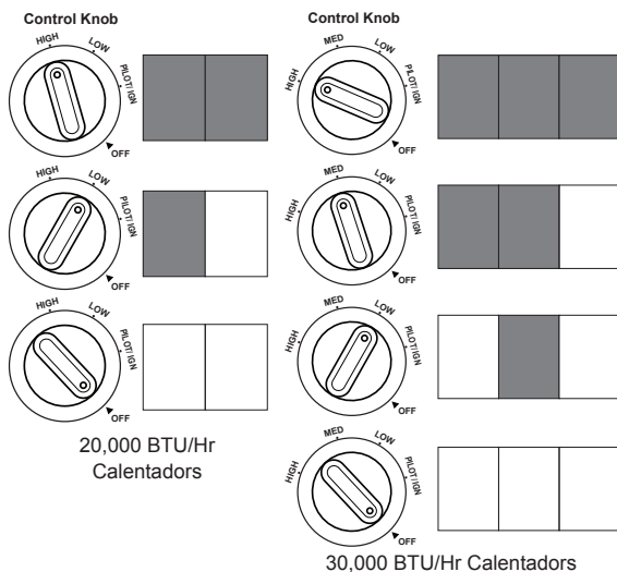
Figure 18 - Patrones de quemador
