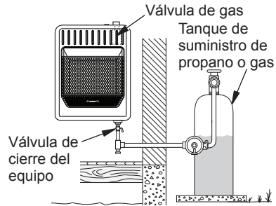
Figura 16 - Propano suministro de gas
