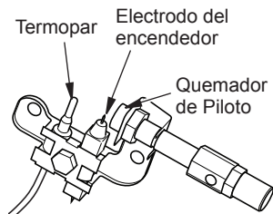
Figure 19 - Conjunto de piloto
