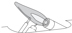
Figura 23 - Patrón correcto de la llama del piloto
