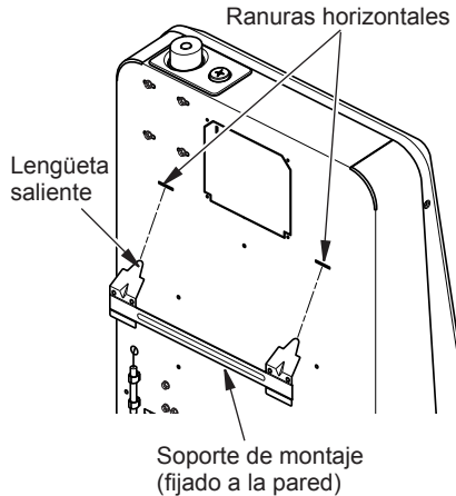
Figura 10 - Montaje del calentador en el soporte de montaje
