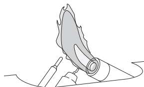
Figura 24 - Patrón incorrecto de la llama del piloto
