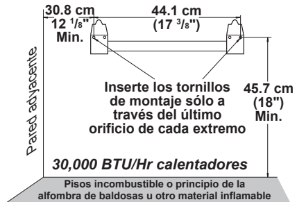
Figura 7 - Distancias mínimas del soporte de montaje
