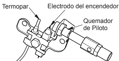
Figura 21 - Conjunto de piloto
