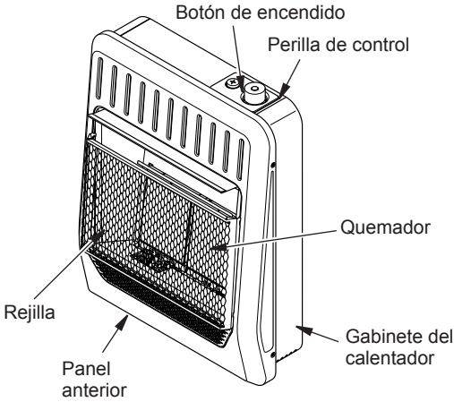
Figura 1 - Calentador de gas sin ventilación
