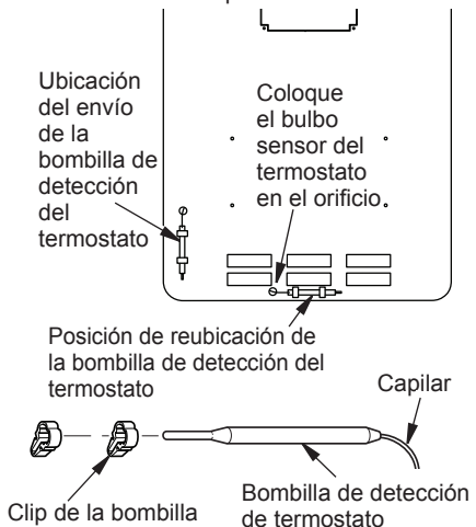
Figura 6 - Bombilla de detección del termostato móvil
