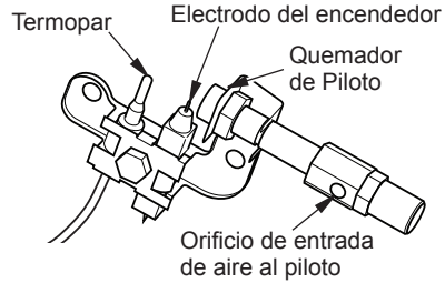
Figura 27 - Orificio de entrada de aire al piloto
