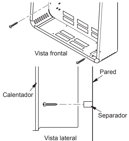
Figura 11 - Instalación de los tornillos de montaje inferiores
