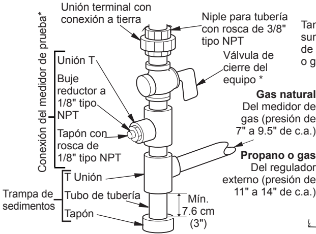
Figura 12 - Conexión de gas
