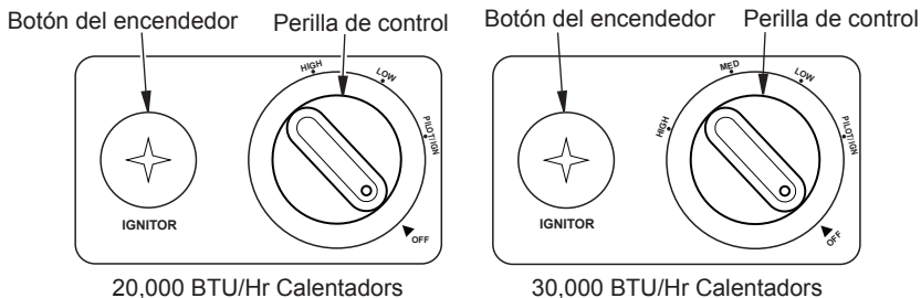
Figure 17 - Perilla de control en la posición OFF (apagado)
