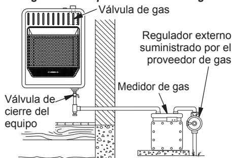
Figura 17 - Suministro de gas natural
