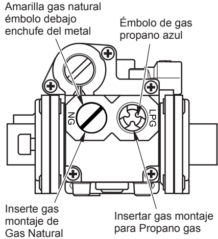
Figura 12 - Regulador de Gas
