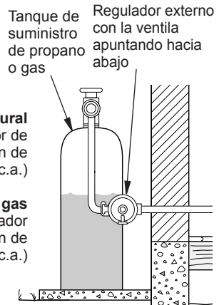
Figura 14 - Regulador externo con la ventila apuntando hacia abajo (sólo propano y gas)
