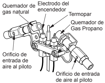
Figura 19 - Conjunto de piloto
