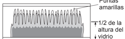
Figura 23 - Patrón incorrecto de la flama del quemador
