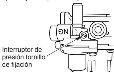
Figura 25 - Interruptor de presión del regulador de gas
