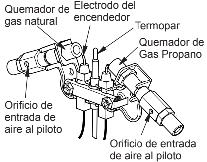
Figura 24 - Orificio de entrada de aire al piloto
