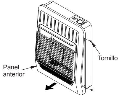
Figura 5 - Desmontaje del panel anterior
