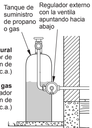
Figura 17 - Regulador externo con la ventila apuntando hacia abajo (sólo propano y gas)
