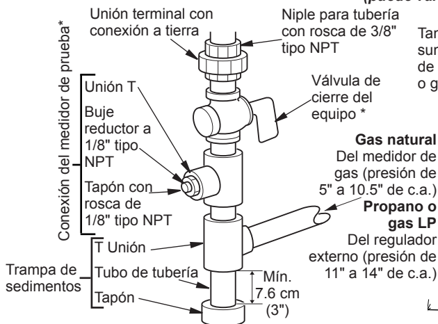
Figura 13 - Conexión de gas
