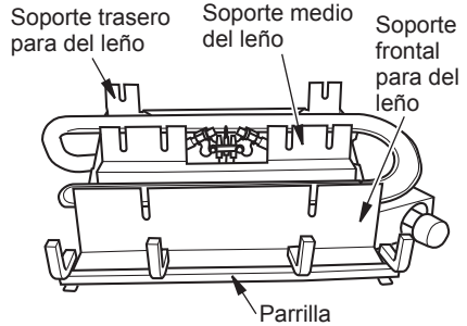
Figura 18 - Asamblea base del calentador
