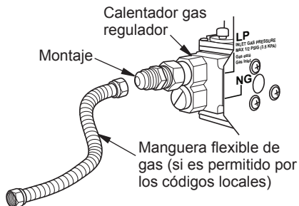
Figura 12 - Colocación flexible manguera de gas al calentador regulador de gas (puede variar de la ilustración)
