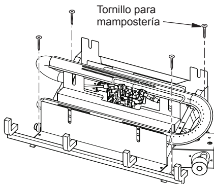
Figura 10 - Instalación del conjunto de la base en el suelo de la chimenea
