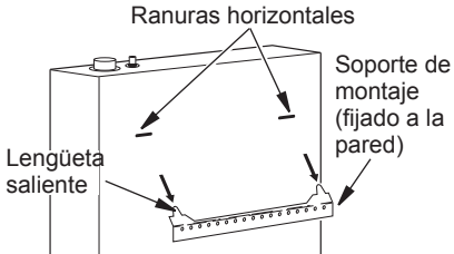
Figura 12 - Montaje del calentador en el soporte de montaje
