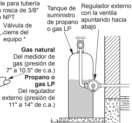
Figura 15 - Regulador externo con la ventila apuntando hacia abajo (sólo propano y gas LP)
