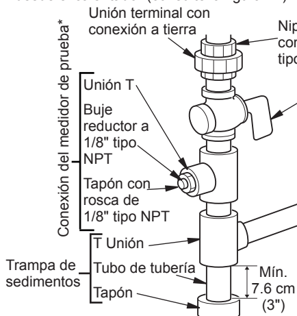
Figura 14 - Conexión de gas
