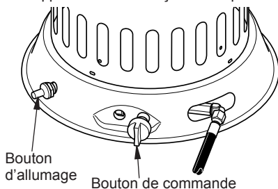
Figure 5 - 80 000 BTU Controls ARRÊT DE L'APPAREIL
