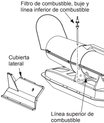
Figura 11 - Desmontaje del filtro de combustible
