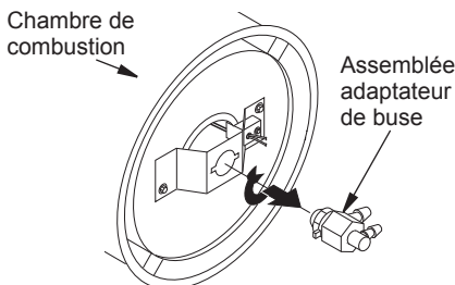
Figure 15 - Retrait de assemblée adaptateur de buse
