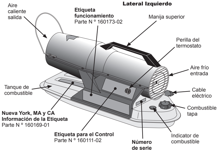
Figura 2 - Identificación del producto y ubicación de las etiquetas
