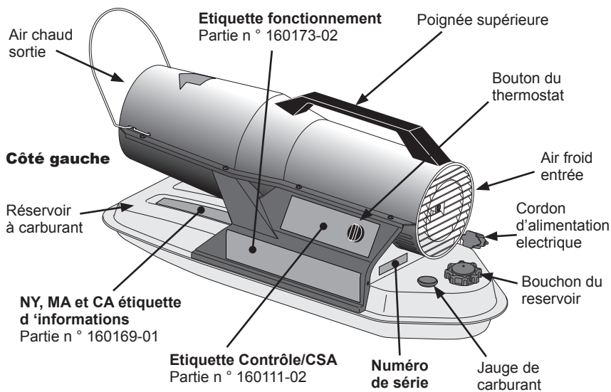
Figure 4 - Identification du produit et emplacement des étiquettes
