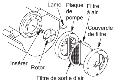
Figure 7 - Localisation du rotor
