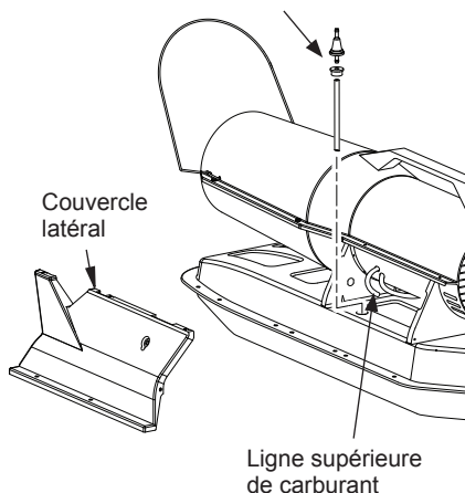
Figure 11 - Retrait du filtre de carburant
