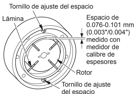
Figura 18 - Ubicaciones del tornillo de ajuste del espacio
