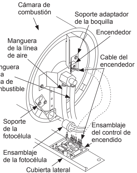
Figura 12 - Desconexión de los cables del encendedor del ensamblaje del control de encendido
