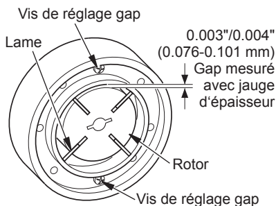
Figure 18 - Emplacements gap vis de réglage
