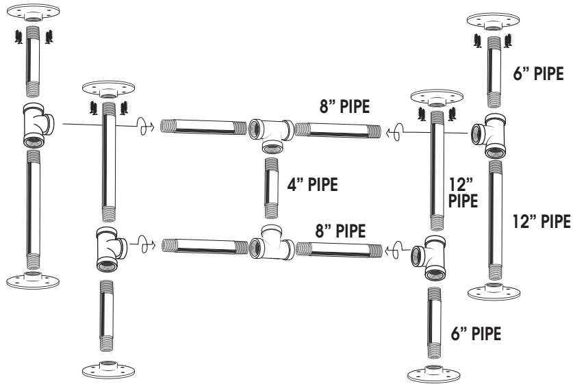
B - 6 X TEES
