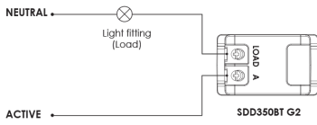
SDD350BT G2 - Optional wiring diagram
