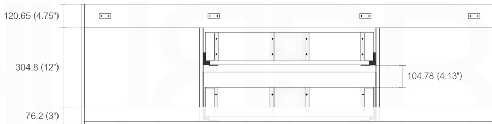
. TOP ELEVATION
