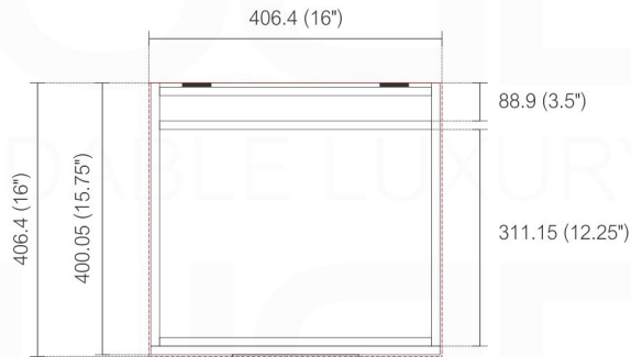
. TOP ELEVATION
