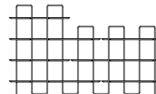
MODULES 03 + 05 + U dimensions 301 × 176,3 × 39,2 cm
