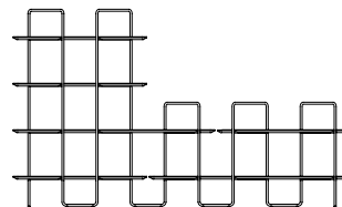
MODULES 03 + 04 + U dimensions 301 × 176,3 × 39,2 cm
