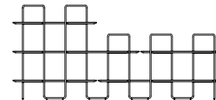
MODULES 02 + 04 + U dimensions 301 × 134,8 × 39,2 cm
