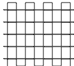
BASIC MODULE 12 dimensions 238 × 217,9 × 39,2 cm
