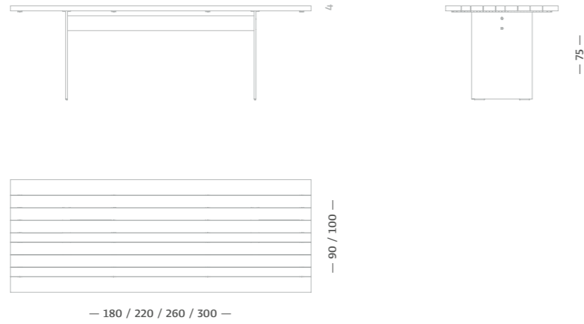
SC 41 Outdoor Tisch / Table
