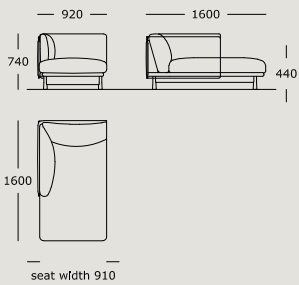
Module 7 Chaise long, left arm
