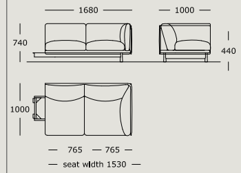
Module 6 Side module, right arm
