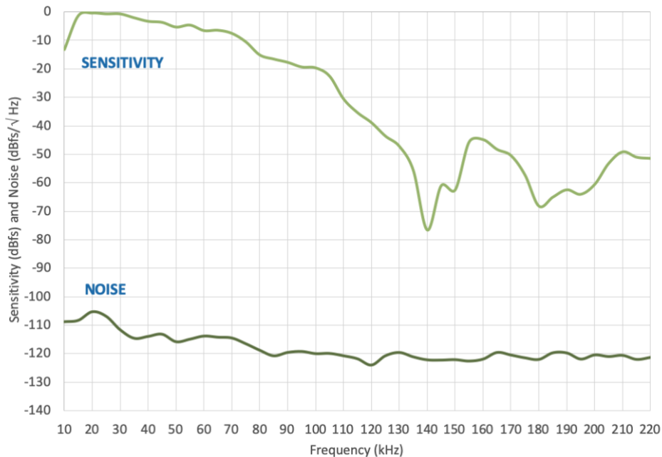
Song Meter Mini Bat Sensitivity and Noise
