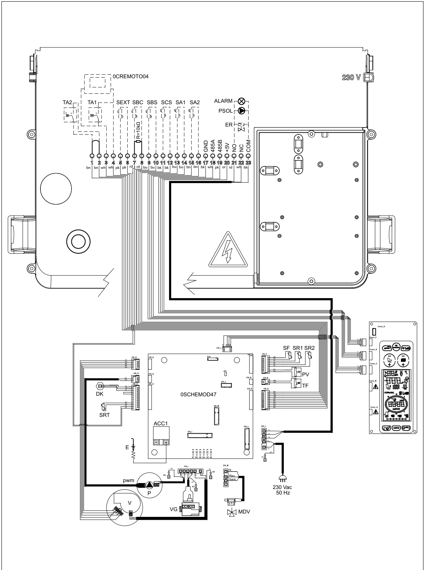
Fig. 32 Esquema eléctrico KRB
