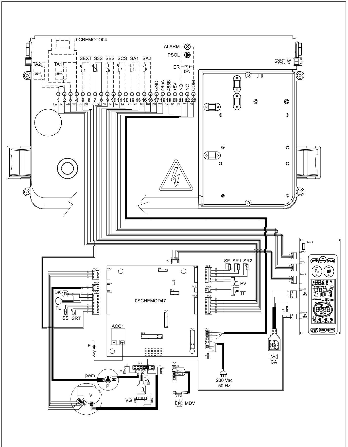
Fig. 24 Esquema eléctrico KC
