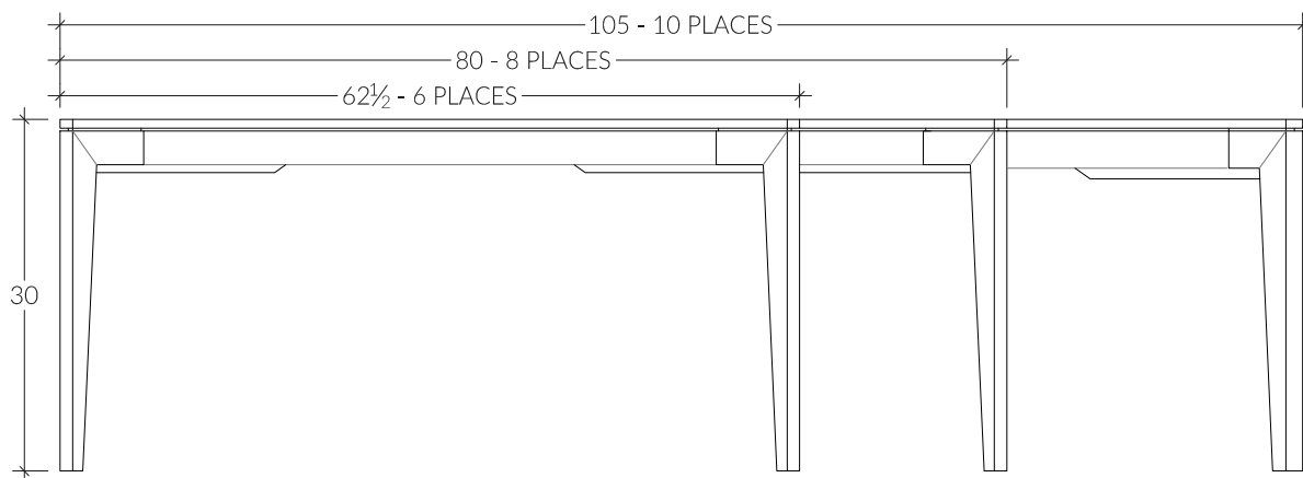
VUE AVANT
