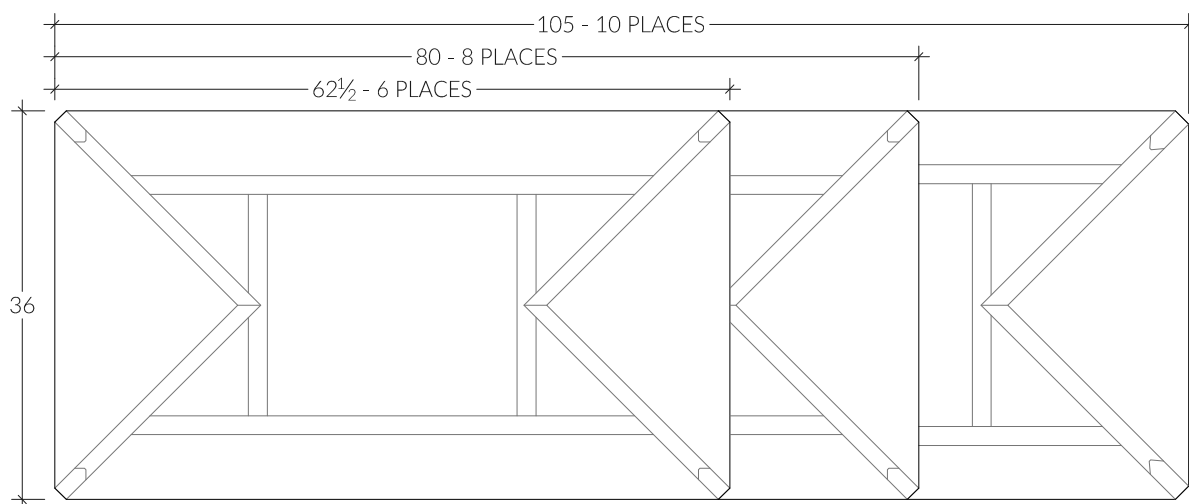
VUE PLAN
