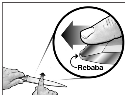
Figura 3. Obtención de una rebaba definida a lo largo del filo del cuchillo antes del asentado del filo de la etapa 2. Es posible detectar la rebaba si desliza el dedo transversalmente sobre el filo. Precaución! Leer el texto.
