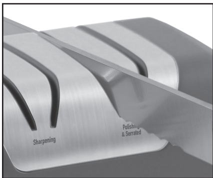
Figura 5. Cuchillo serrado en la etapa 2.
