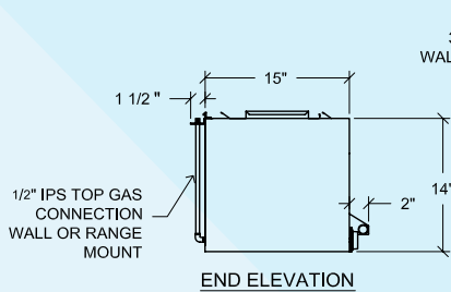
END ELEVATION
