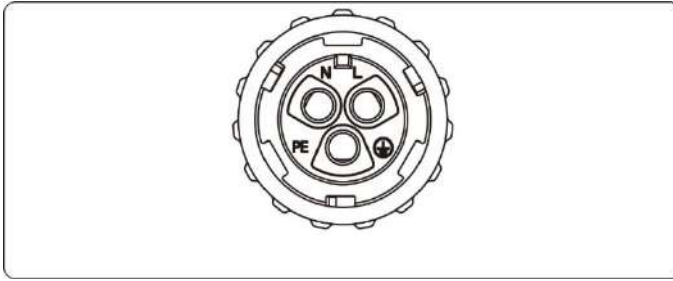
Imagen 5.9 Patrón de conexionado del conector CA
