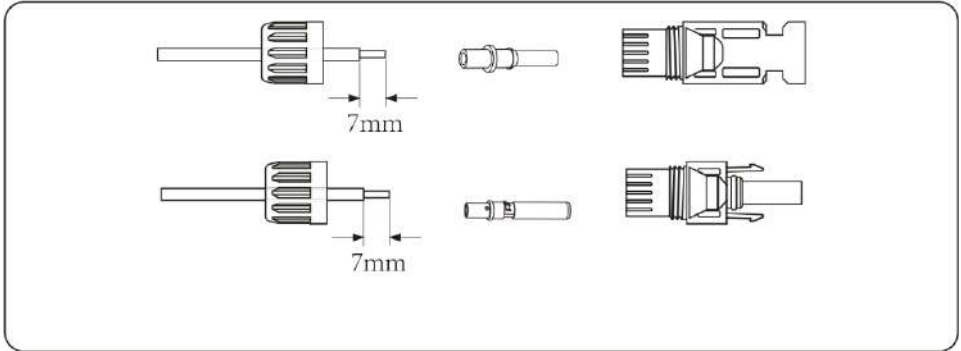
Imagen 5.3 Desmonte la tuerca de tope de conexionado
