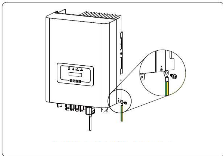
Imagen 5.11 La instalación del tierra de la carcasa.
