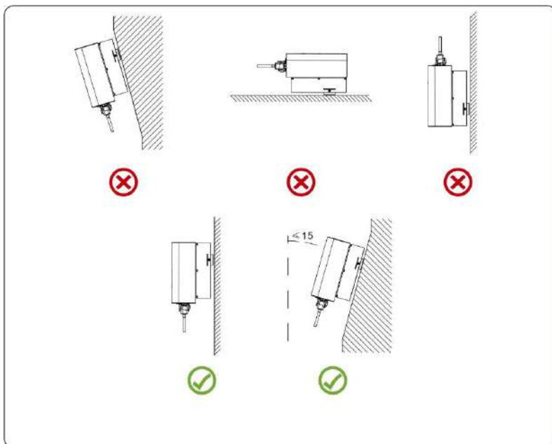
Imagen 4.2 ángulo de instalación
