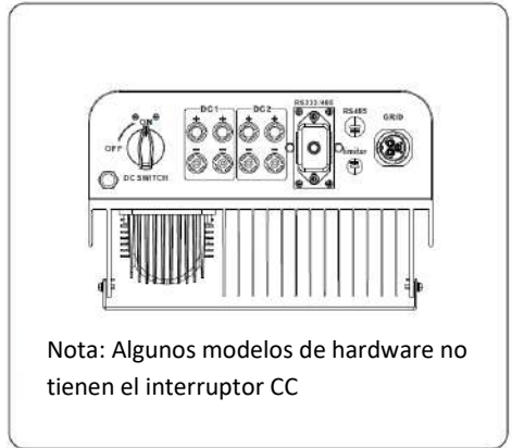
Imagen 1.2 Vista inferior
