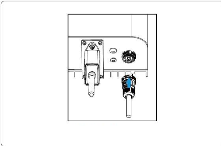
Imagen 5.10 Conexión de la entrada de CA
