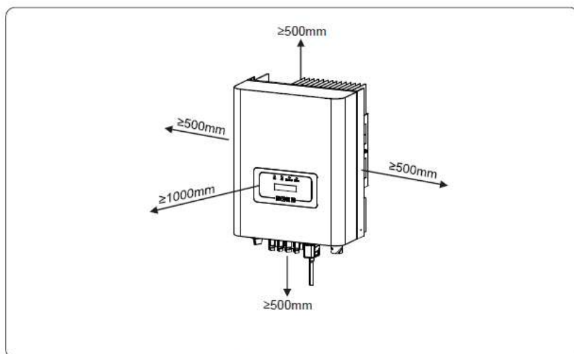
Imagen 4.3 espacio de instalación
