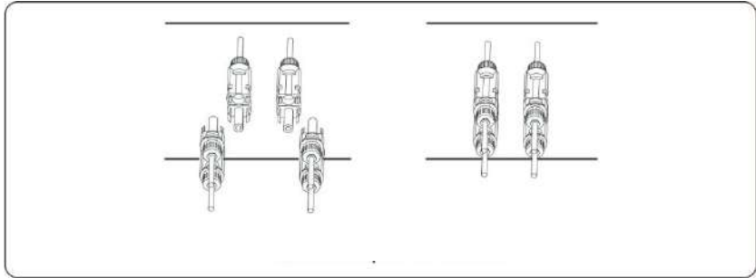
Imagen 5.6 Conexión de las entradas CC
