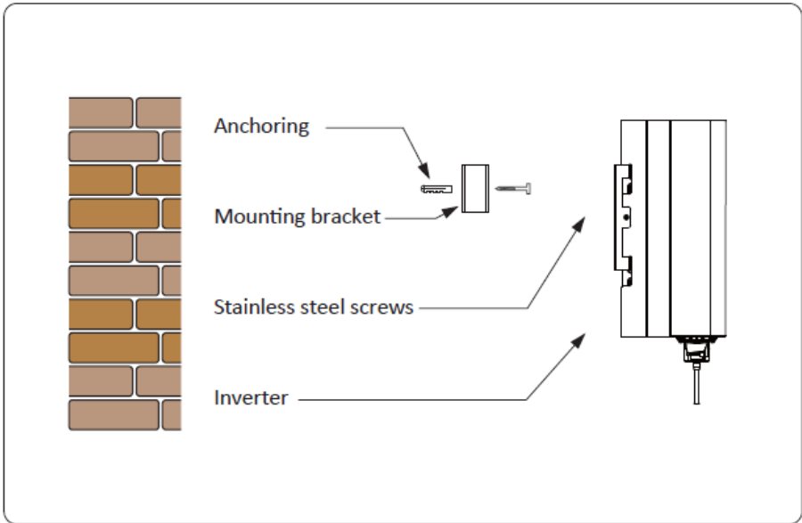
Imagen 4.4 Instalación del inversor
