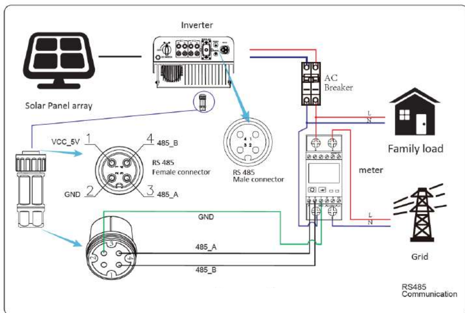
Imagen 7.2 Diagrama de conexión del medidor Maxge SGM230M
