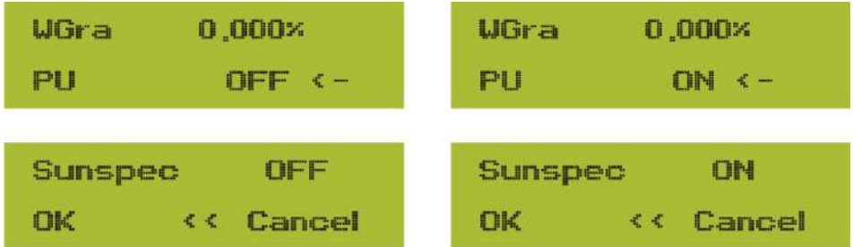
Imagen 8.30.3 Caída de potencia activa
