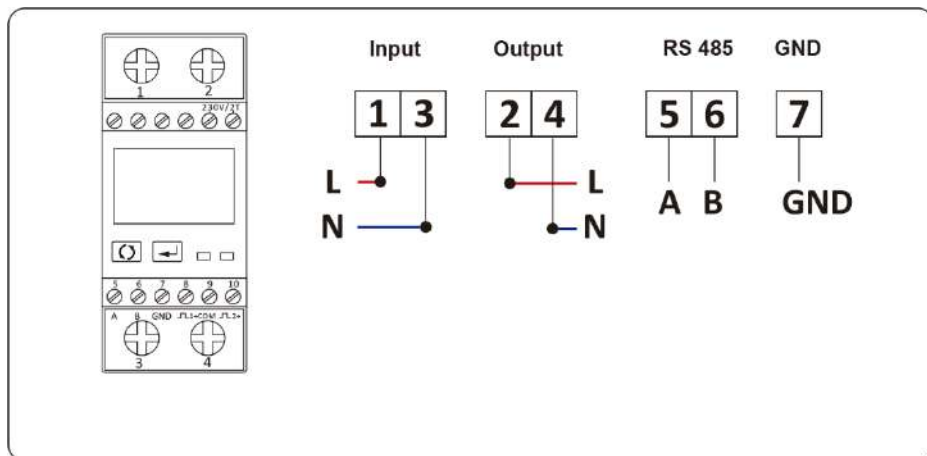
Imagen 7.1 Medidor Maxge SGM230M
