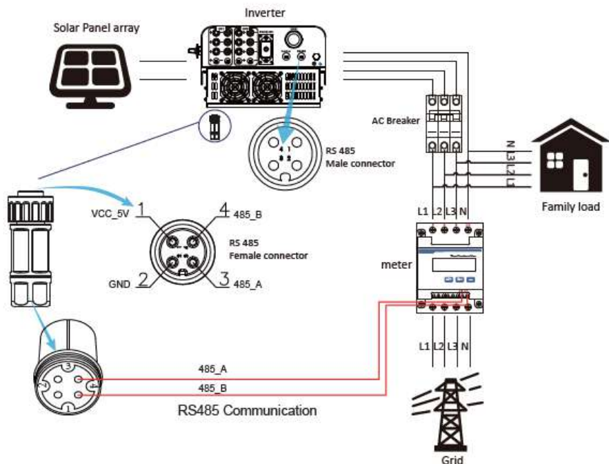
Imagen 7.6 Diagrama de conexonado de medidor REMTCHNTTP
