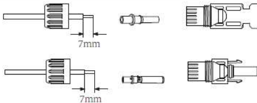
Imagen 5.3 Desmonte la tuerca de tope de conexionado
