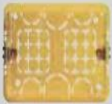
503E (106 × 71 × 52 mm) superficie albañilería
