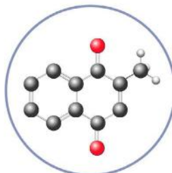
Menadione
