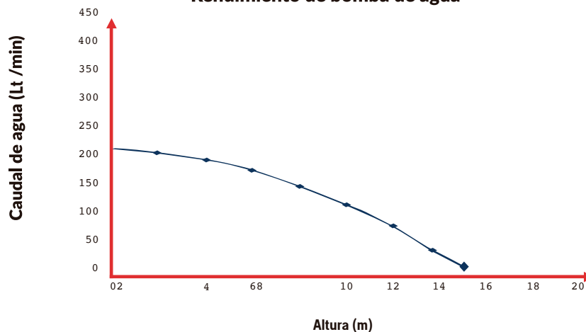
Rendimiento de bomba de agua
