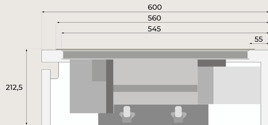
Kastdoorsnede zij-aanzicht
