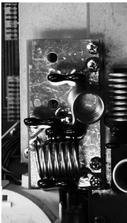
ALS-600
