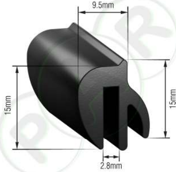
PR135 EPDM Ford Anglia back 1/4 Rubber
