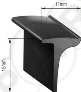
PR275 T - Section
