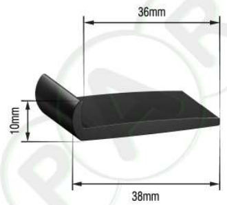
PR1193 EPDM Carpet Edge
