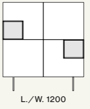
Box Modulo + Box Elle - Cube H. 1104 x P./D. 478
