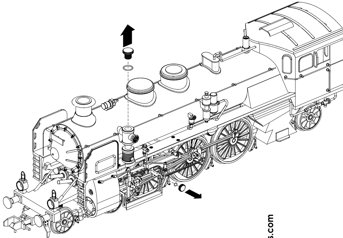
Fig. 8: Deckel abschrauben
