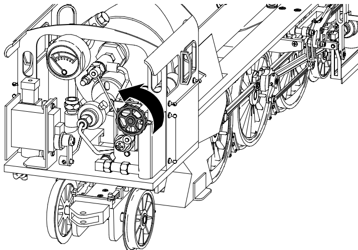
Fig. 16: Gasregler aufdrehen
