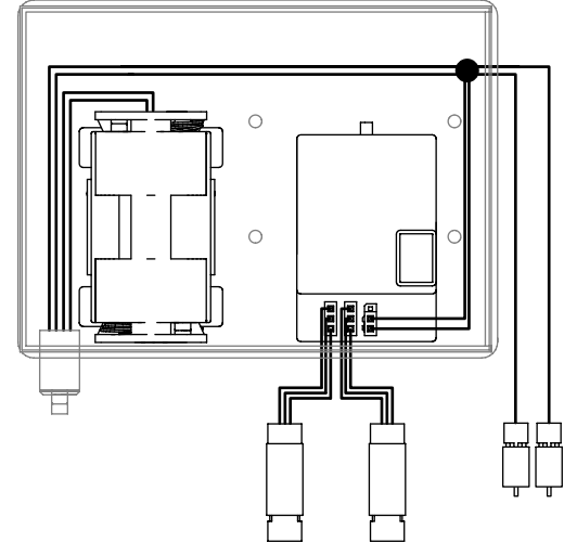
Fig. 1: Anschlussschema
