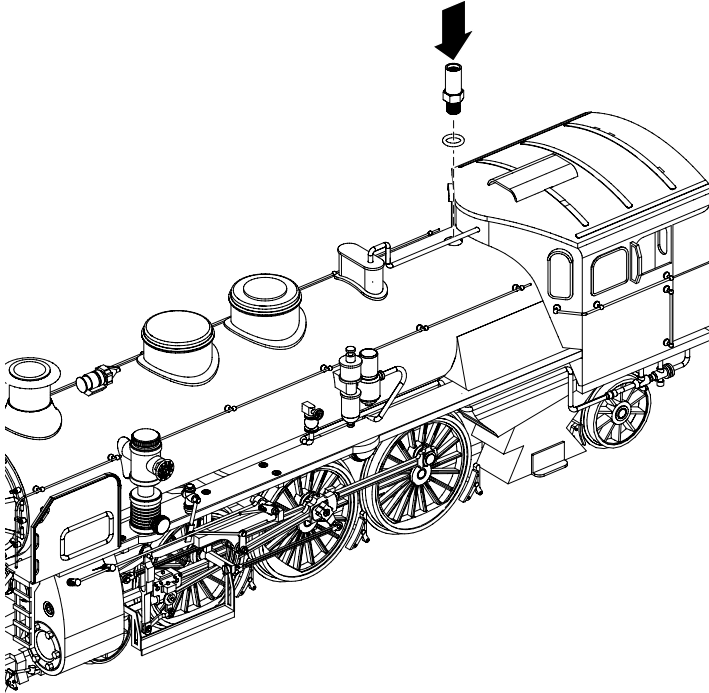
Fig. 11: Sicherheitsventil überprüfen
