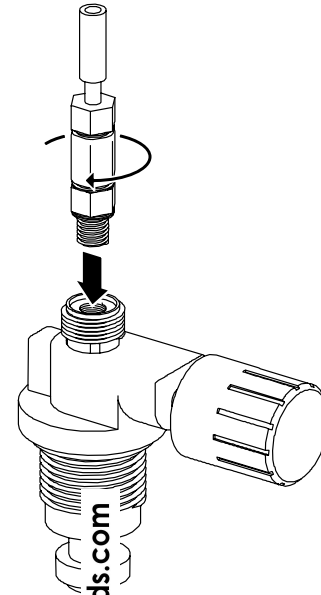
Fig. 13: Gasumfüll-Adapter rieren
