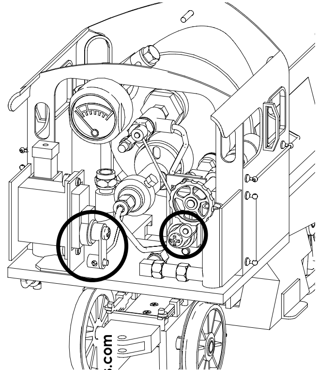
Fig. 22: Servo einstellen
