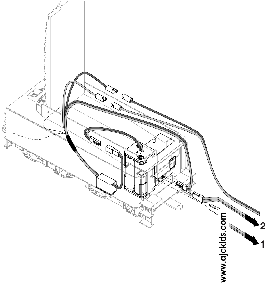
Fig. 4: Servo anschließen
