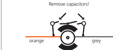
Figure 22: 5-pole Märklin® motor
