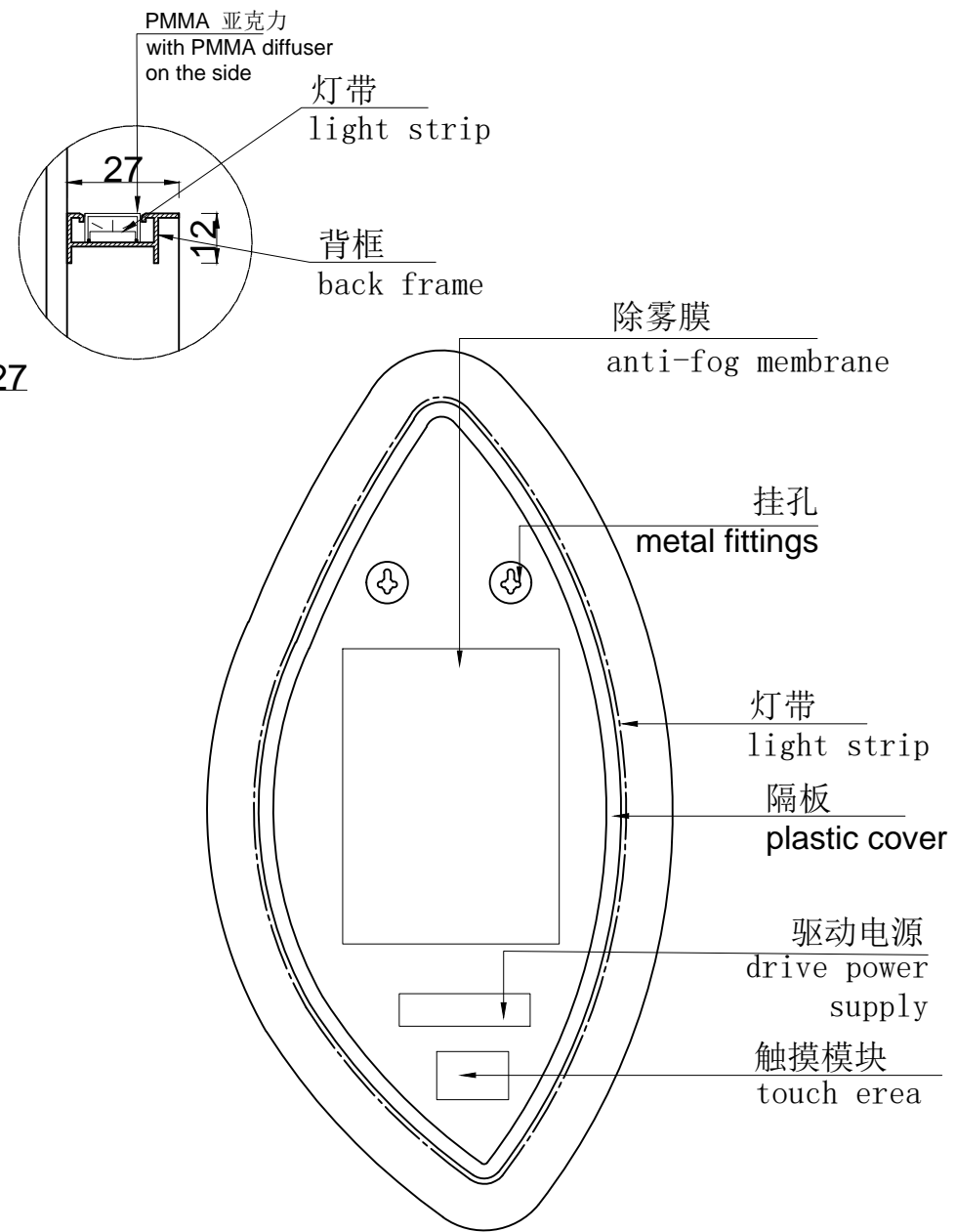
背面 backside
