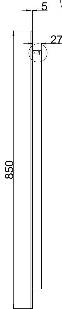
侧面 side
