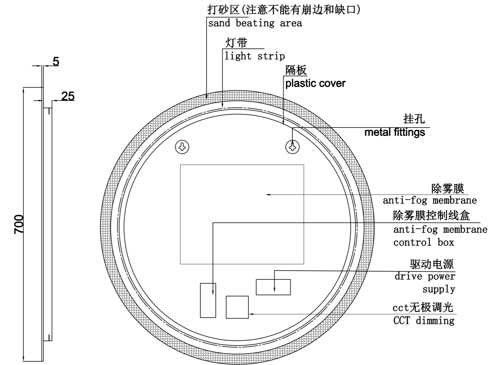
侧面 side
