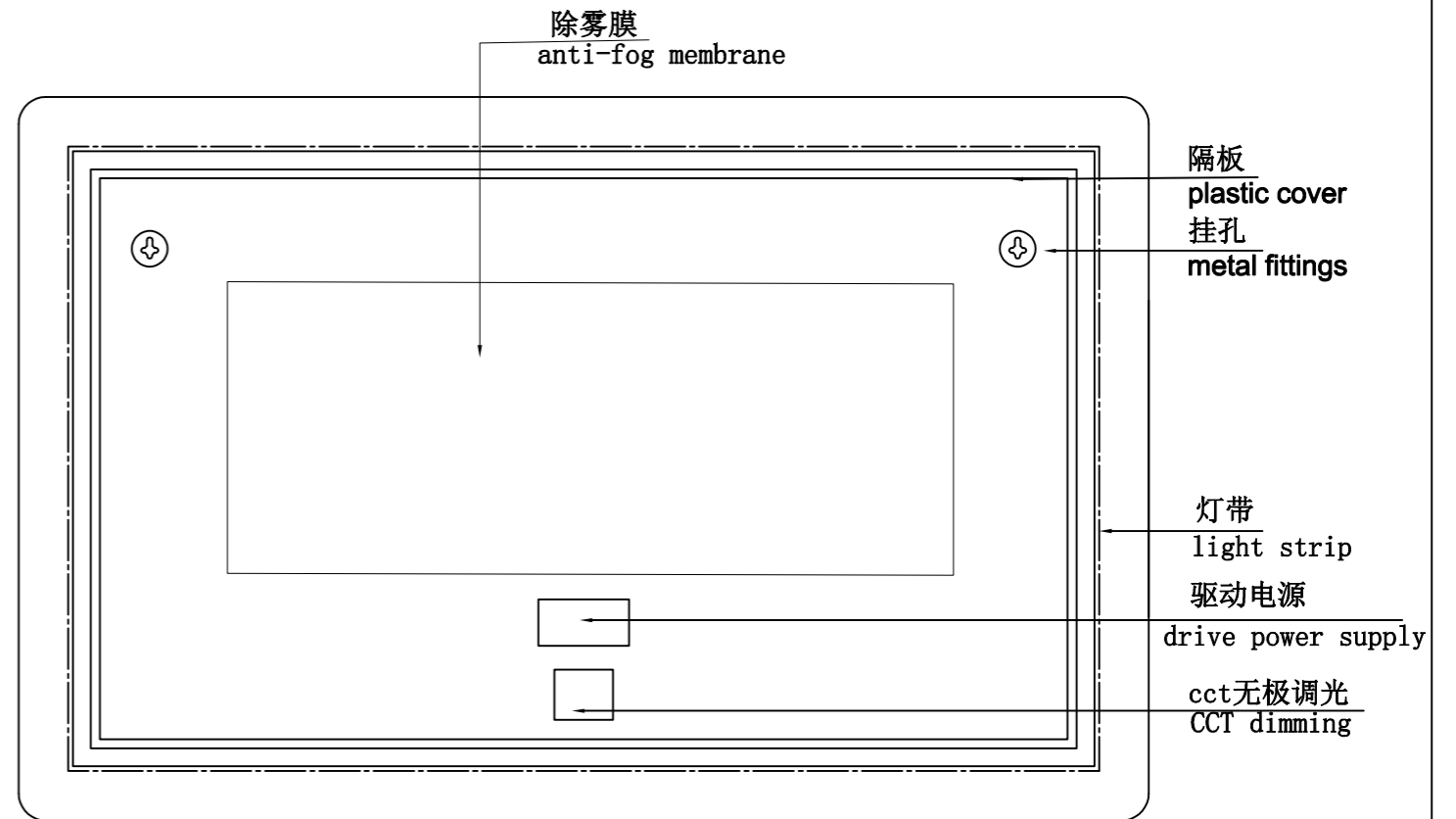
背面 backside
