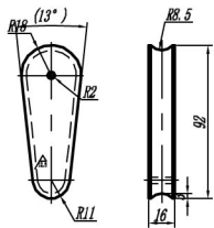
(5) Spring
