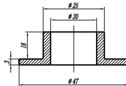
(4) Grommet/ Bushing
