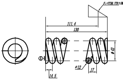
(5) Spring
