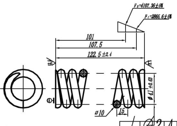
(5) Spring
