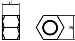
(1) M20 Nut
