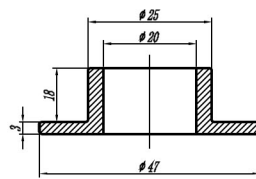
(4) Grommet/ Bushing
