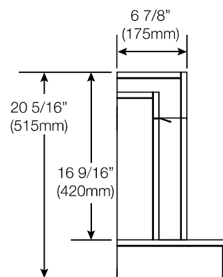
vue latérale
