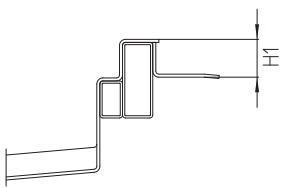
AF Attachment flange 11)
