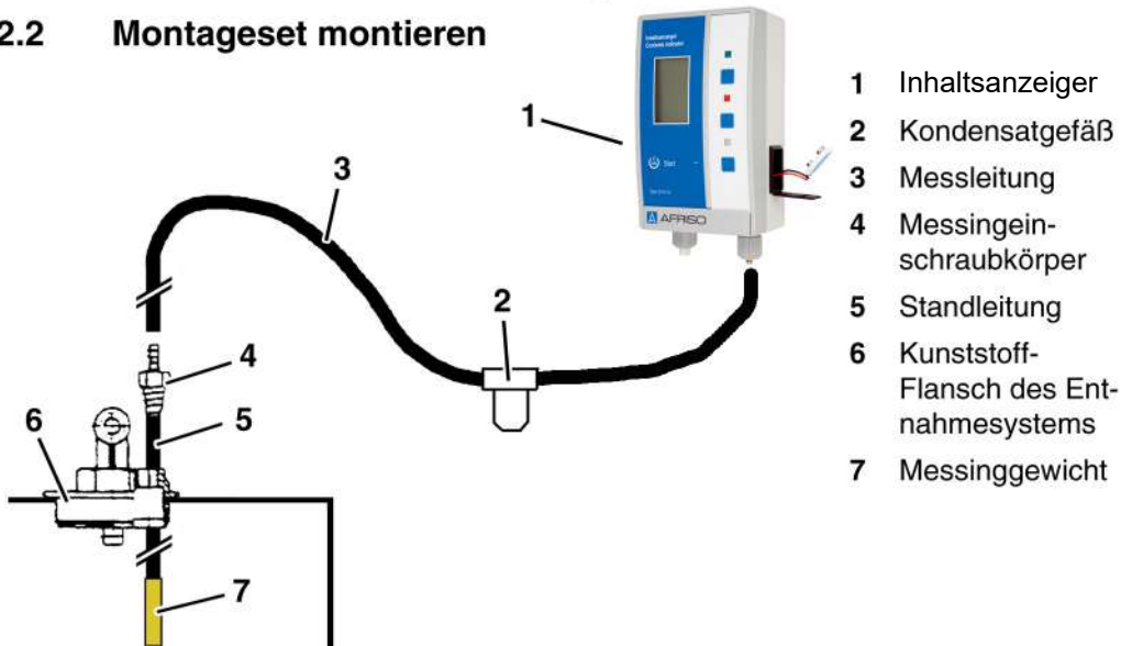
Bild 2: Sofortmontage
